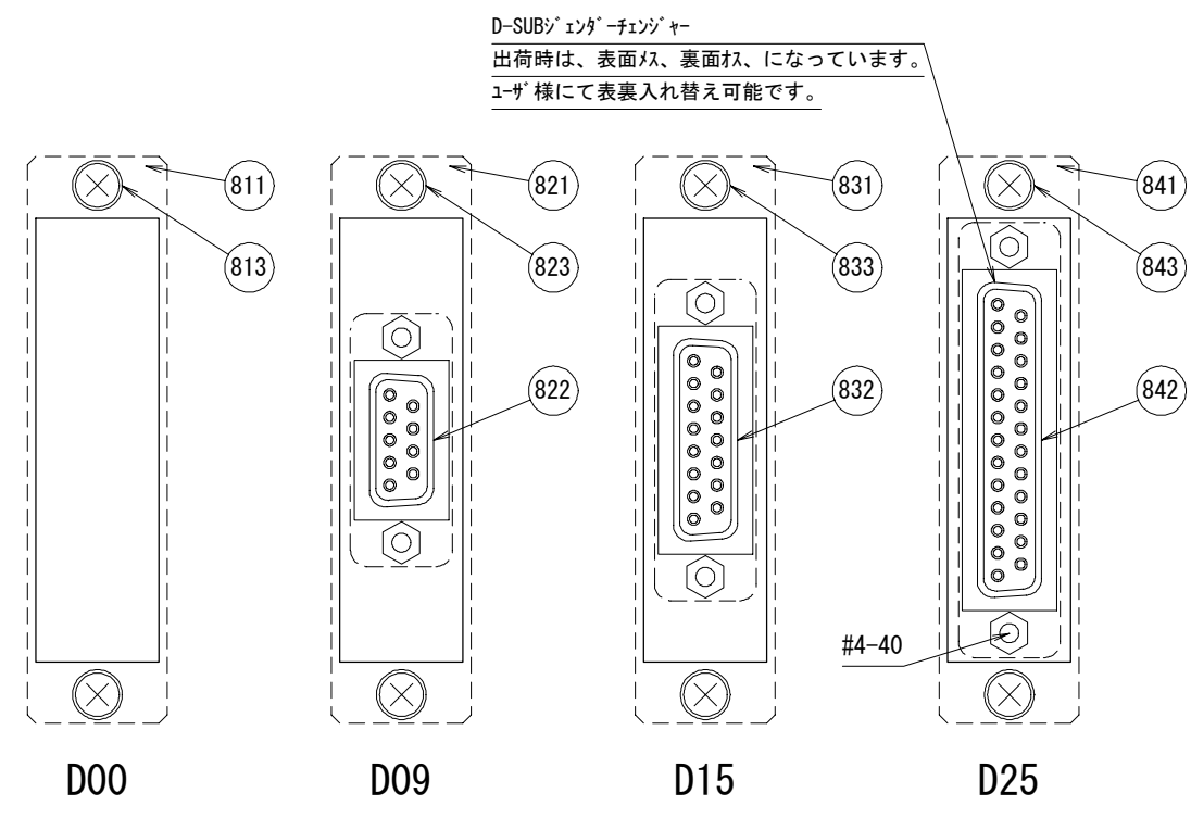
⑧DSUB詳細
