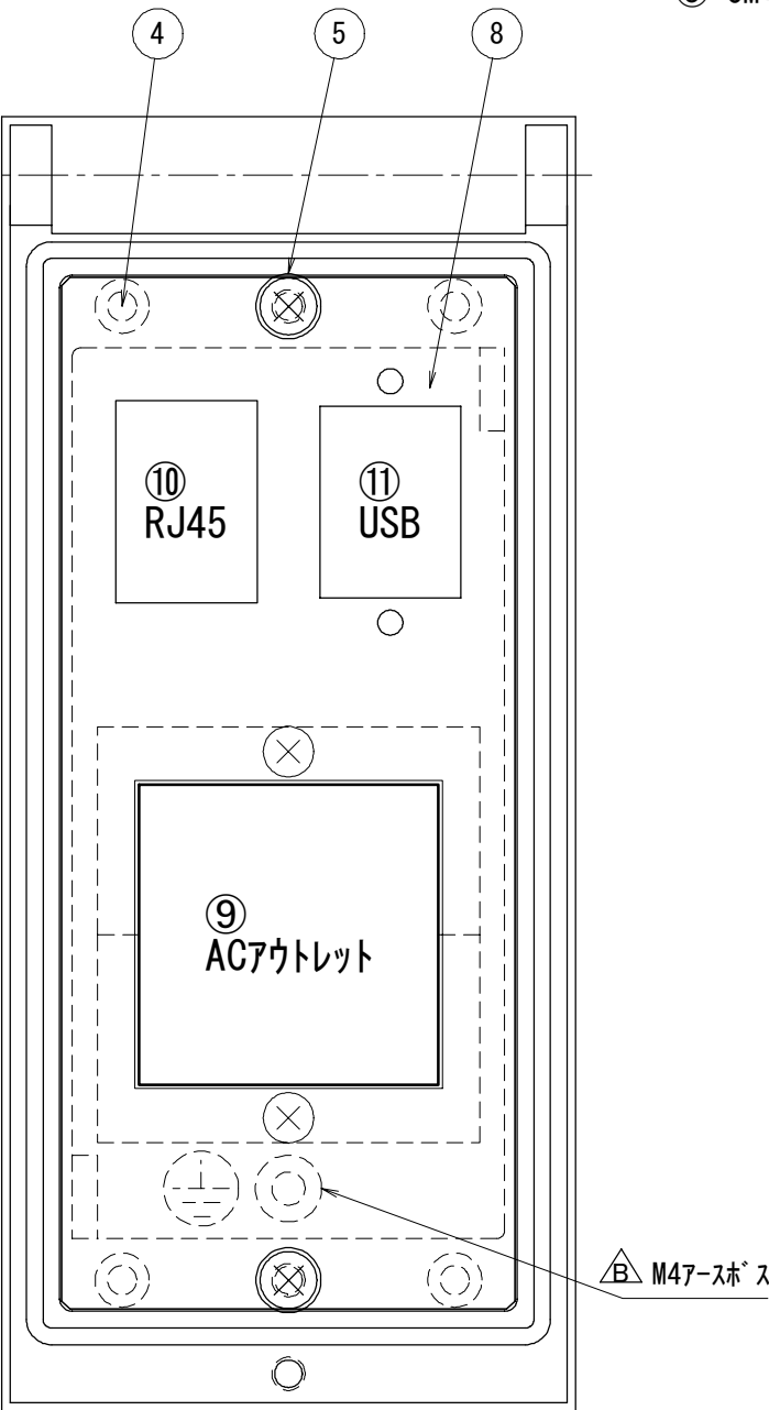
内部図
