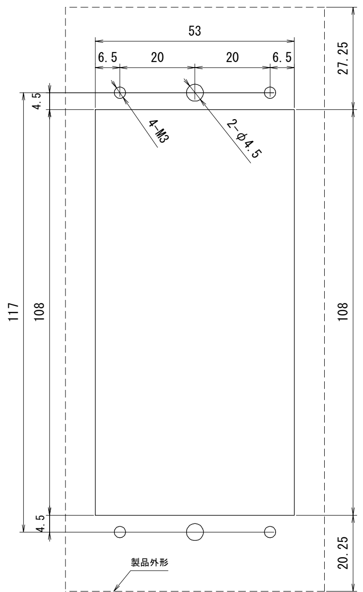
パネルカット図 推奨板厚 t=1.6以上
