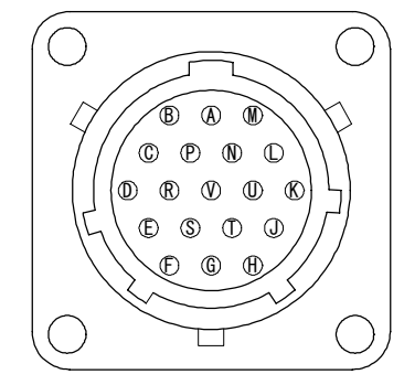
参考図(1.5/1尺) コネクタ嵌合面
