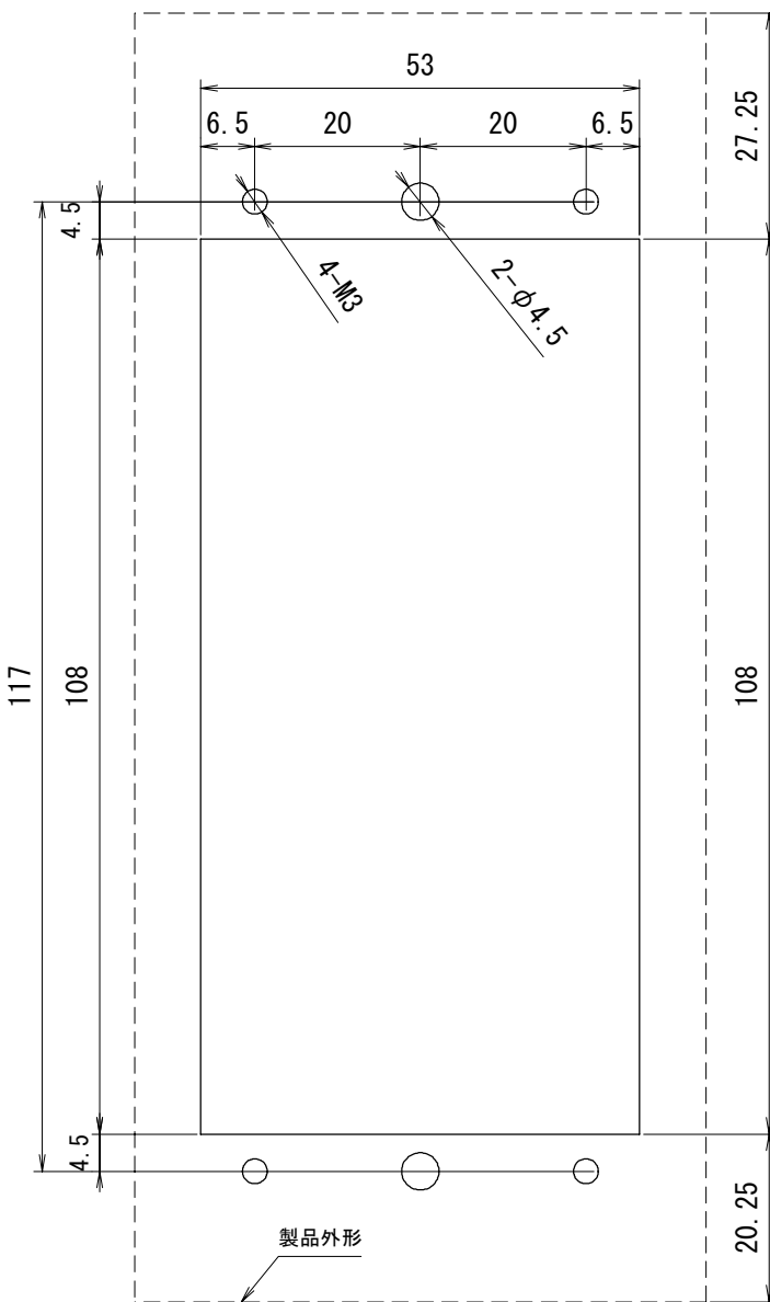
パネルカット図 推奨板厚 t=1.6以上
