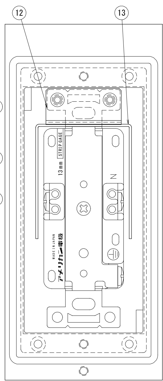
裏面図
