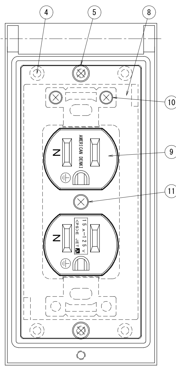
内部図
